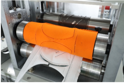
切刀轮装置
