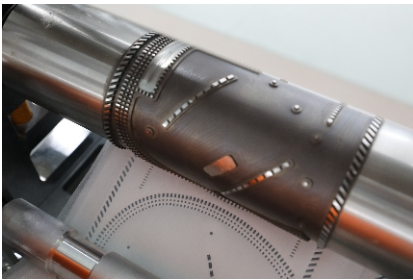
压花轮装置
